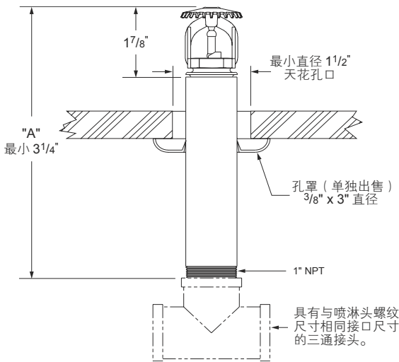
标准 / 快速反应干管上喷式——V3601、V3602
