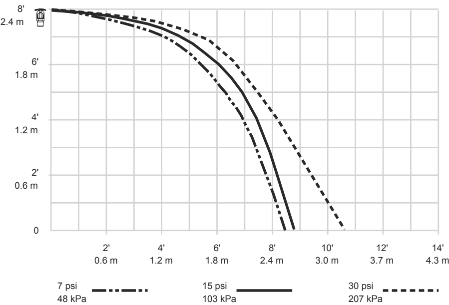
型号 V3601、V3602 K5.6 标准 / 快速反应干管上喷式分布模型——轨迹线
