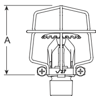
V27 型防护罩 (上喷式或下喷式)
