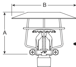
V27 型中间层上喷式
