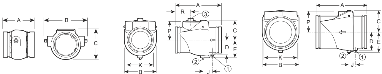
典型 2½ - 3"/65 - 80 毫米阀门 典型 4 - 8"/100 - 200 毫米阀门 ① 1½" NPT 上游排水口 ② 1½" NPT 下游排水口 ③ 2" NPT 排水口 (选配) 典型 10 - 12"/250 - 300 毫米阀门 ① 1½" NPT 上游排水口 ② 1½" NPT 下游排水口
