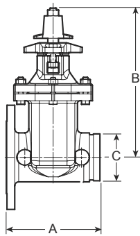
772F 系列暗杆闸阀（沟槽 X 法兰）
