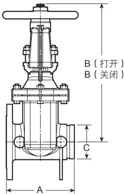
771F 系列明杆闸阀（沟槽 X 法兰）
