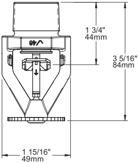
标准上喷式——LP-46 (SIN V4603)
