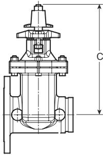
772F 系列暗杆闸阀（沟槽 X 法兰）
