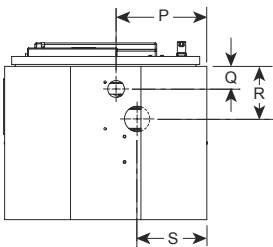
底视图 仅限 1 1/2 - 2 3/4 - 50 mm 尺寸
