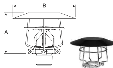
V34 型中间层上喷式
