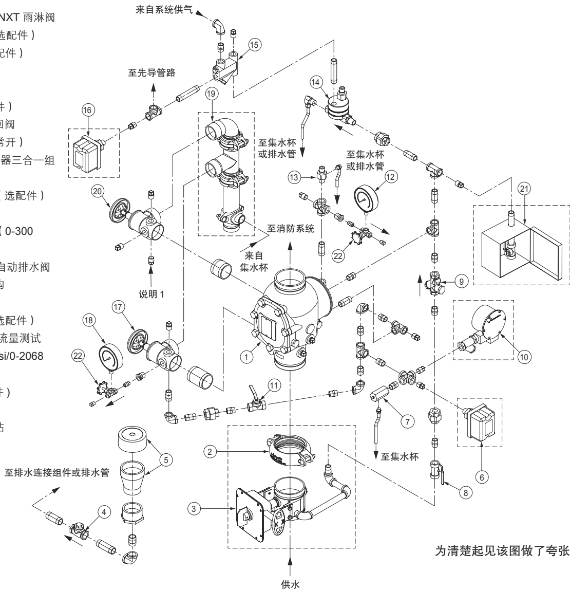
说明 1：75D 系列水柱装置套件连接点。
