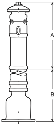
774 系列立式位置指示仪
