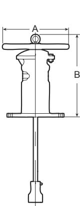
773 系列壁式位置指示仪
