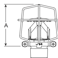
V34 型防护罩 (上喷式或下喷式)
