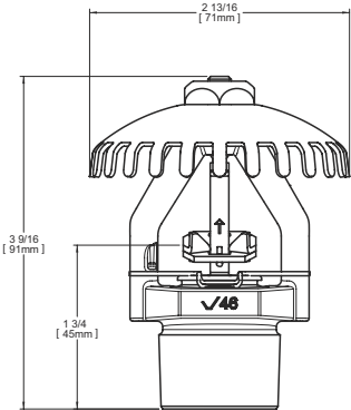
标准上喷式——LP-46 (SIN V4603)
