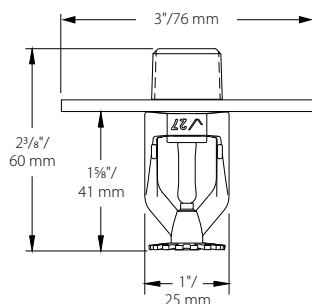
Intermediate Pendant – V2723, V2724
