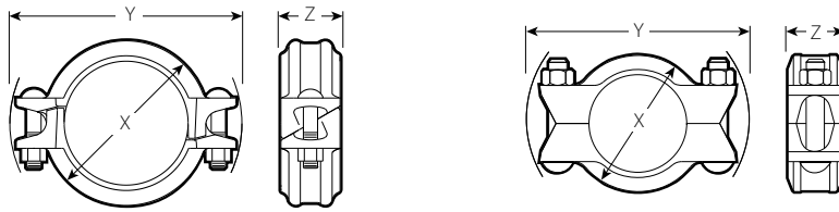
1 ½ – 4\"/&gt;
